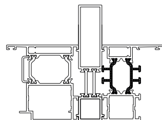
Accouplement de châssis avec profil renforcé
