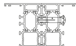
Accouplement de châssis avec profil standard
